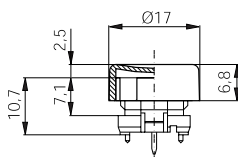
mezera 16 mm 835 000 111
