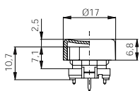
rozteč 16 mm 835 900 013-033
