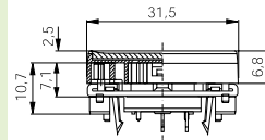
Zmístný 16 mm 835 950 013-033
