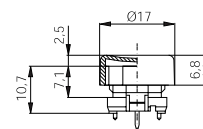
průměr 17 mm
